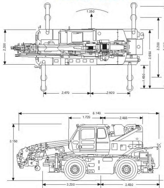
16 Tonne Dimensions
